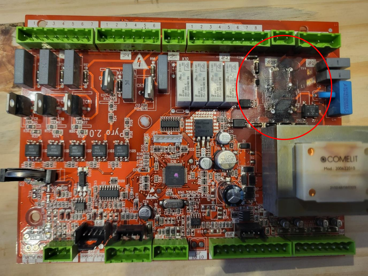
Carte Electronique Pyro – 2.0 – (Après démontage suite deuxième défaut – zone noircie)
