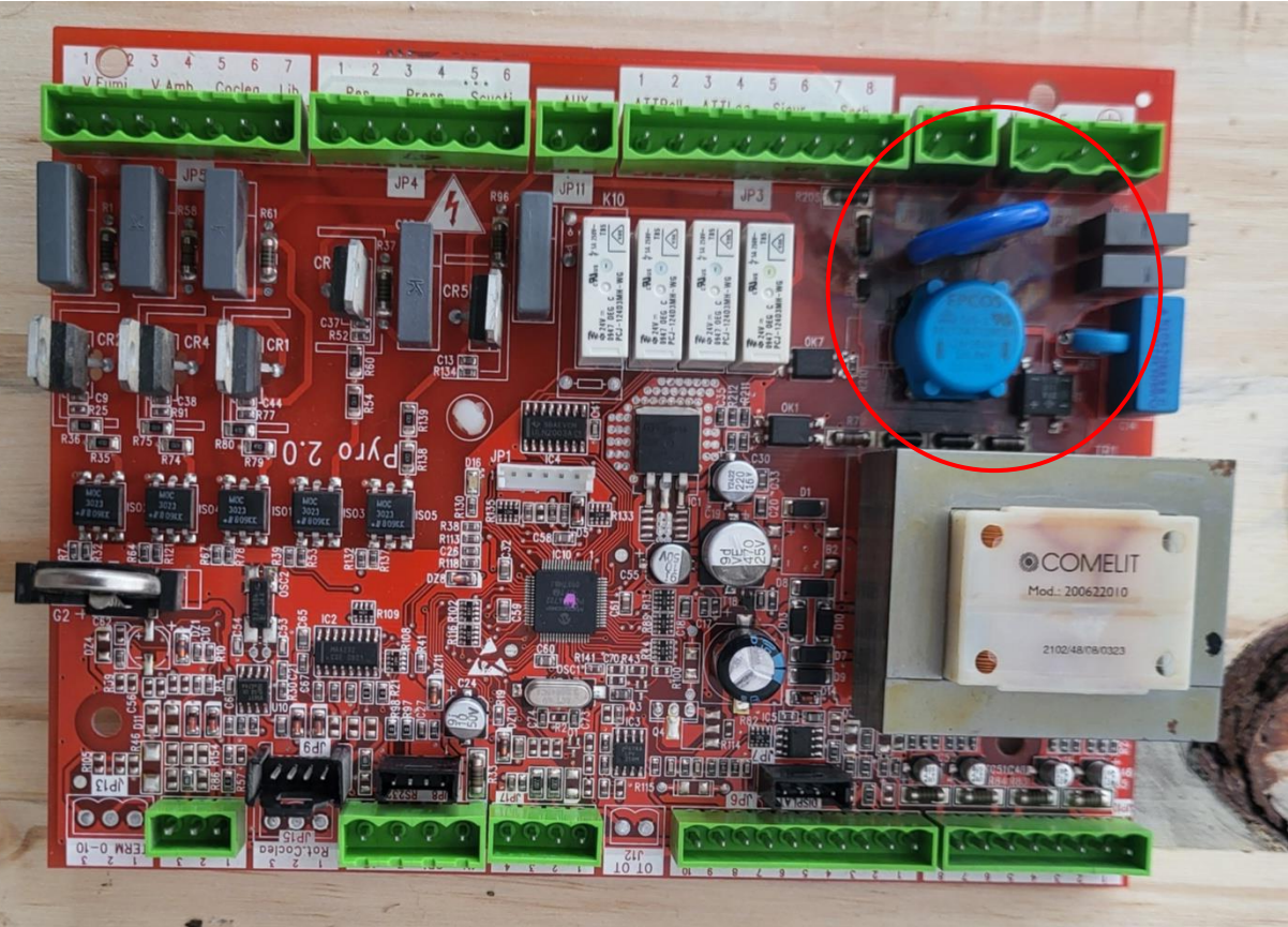
Carte Electronique Pyro – 2.0 – (Après démontage suite deuxième défaut – zone noircie)
