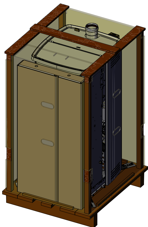
EMBALLAGE EGO AVEC REVÊTEMENT EN ACIER
