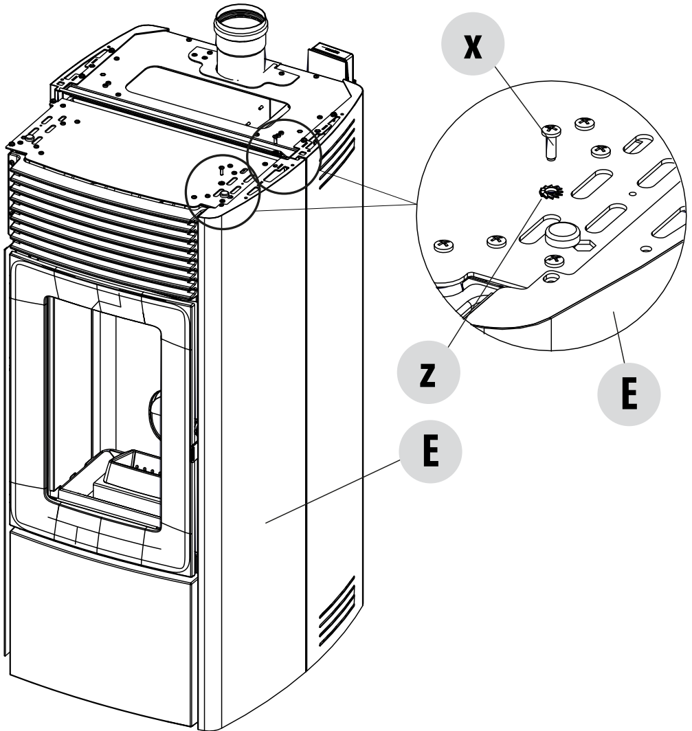
FIXATION SUPÉRIEURE DU PANNEAU EN MÉTAL
