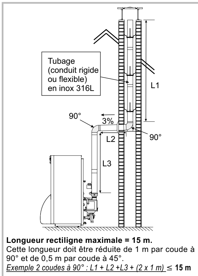
Figure 13 - Possibilité de raccordement B23P
