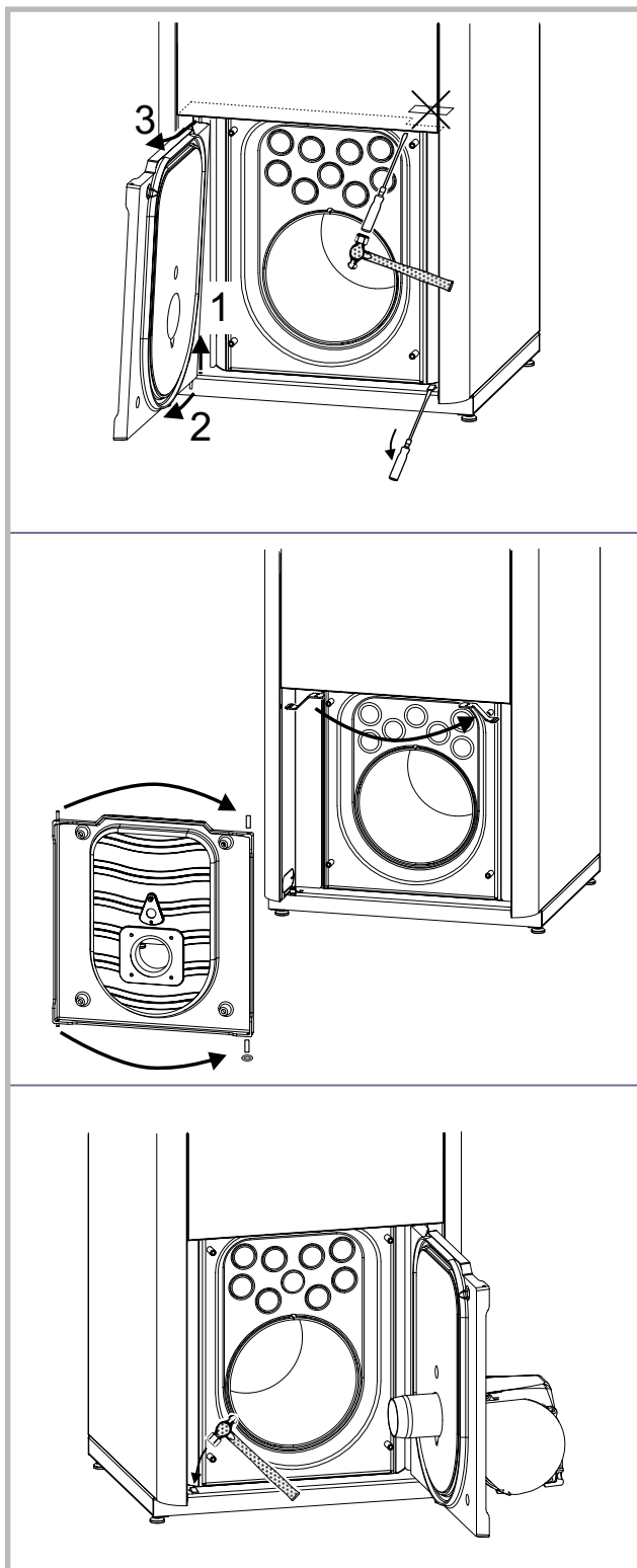
Figure 20 - Porte de foyer réversible
