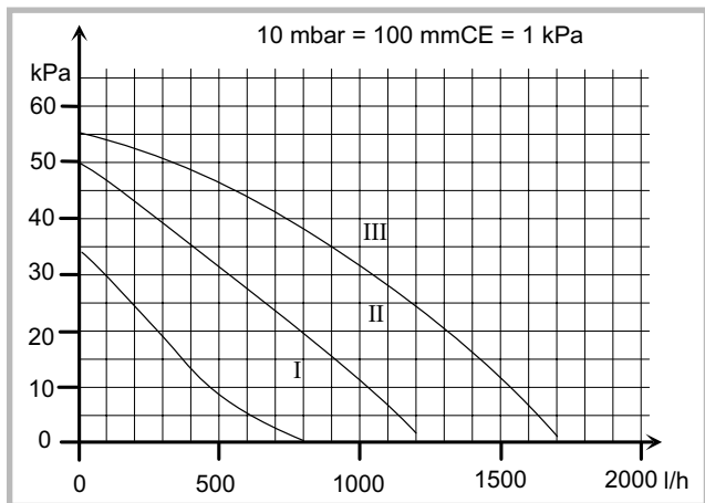
Figure 3 - Pressions et débits hydrauliques disponibles Ambiance Condens 4225
