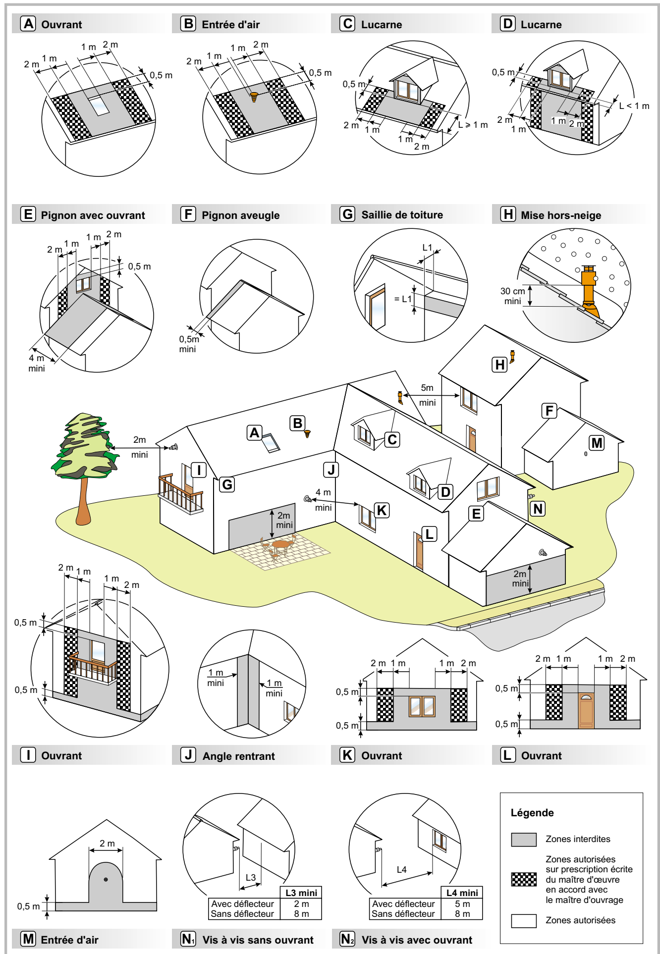
Figure 16 - Règles d'implantation du terminal pour chaudières fioul étanches ≤ 70 kW (C13, C33)
