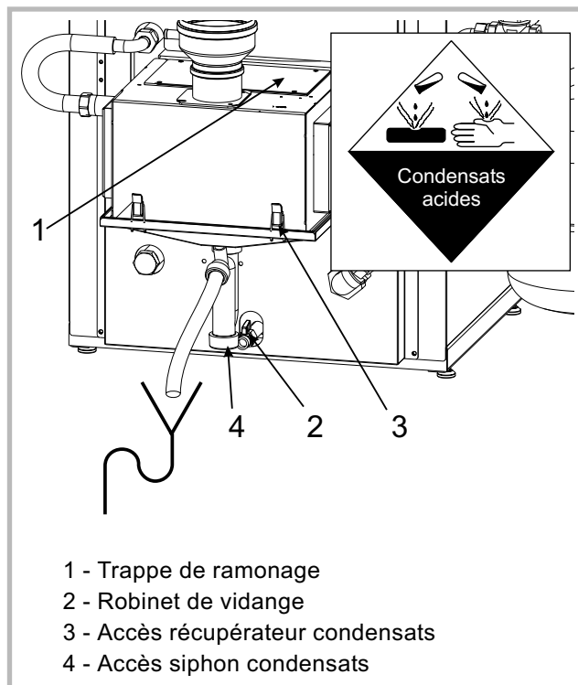
Figure 37 - Arrière de la chaudière
