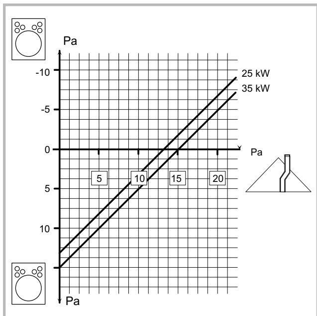
Figure 7 - Pertes de charge du circuit de combustion
