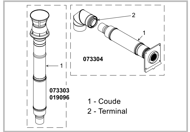
Figure 9 - Éléments des colis ventouse
