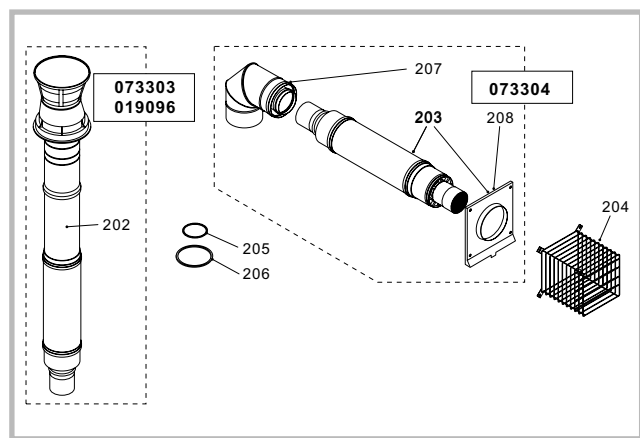
Figure 46 - Vue éclatée (ventouse)
