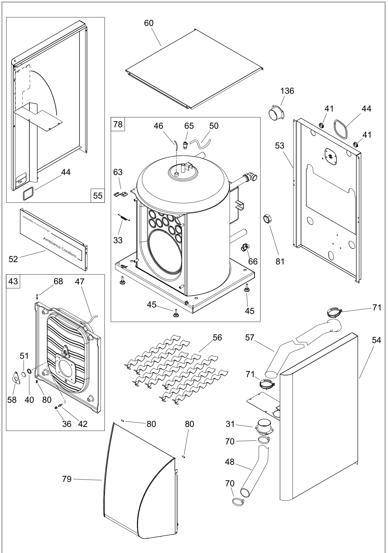
Figure 47 - Vue éclatée (chaudière)
