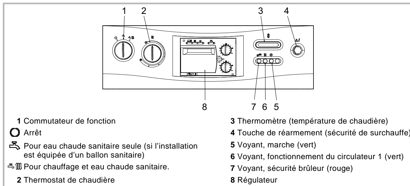
Figure 11 - Tableau de contrôle
