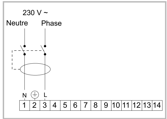
Figure 28 - Protection différentielle
