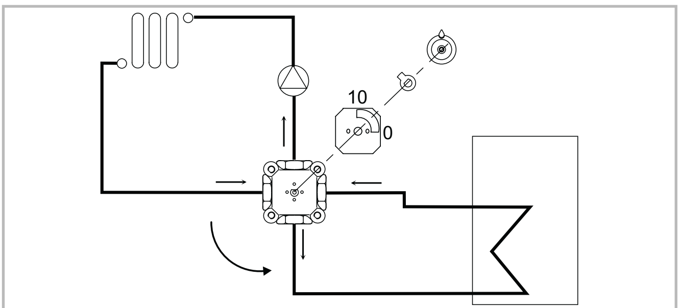
Figure 22 - Montage de la vanne mélangeuse à gauche de la chaudière
