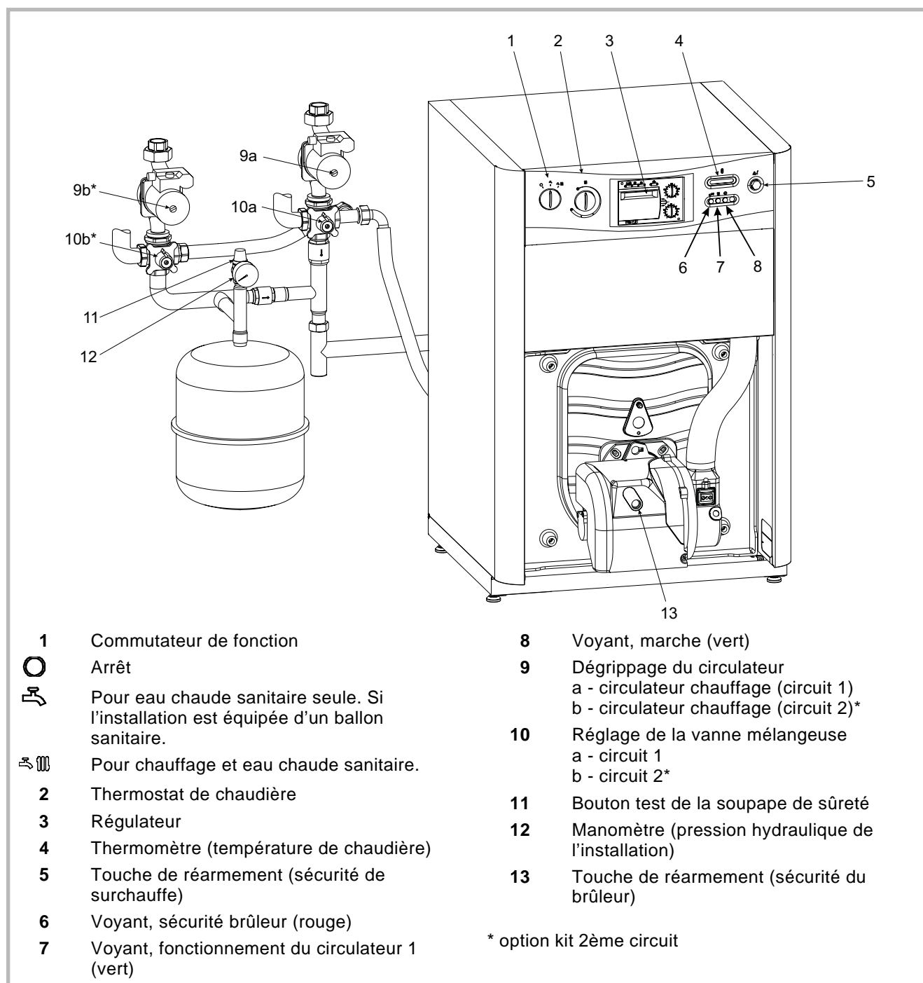
Figure 38 - Organes de commande et de contrôle
