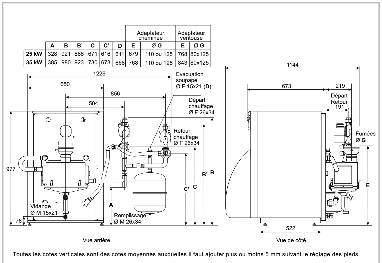
Figure 2 - Dimensions en mm (option kit 2 ème circuit)
