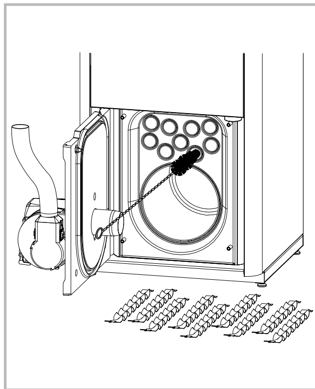
Figure 36 - Accès aux carnaux de l'échangeur
