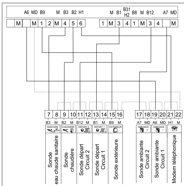
Figure 27 - Câblage du faisceau faible tension
