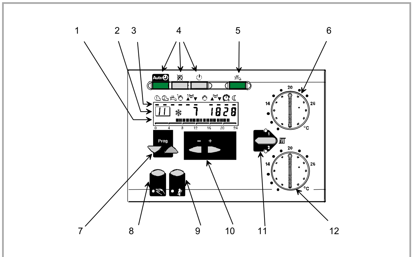
Figure 39 - Touches de fonction du régulateur
