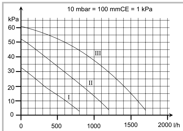
Figure 4 - Pressions et débits hydrauliques disponibles Ambiance Condens 4235
