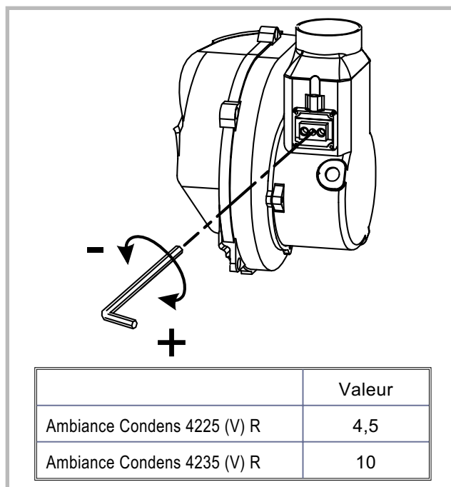
Figure 34 - Réglage du volet d'air
