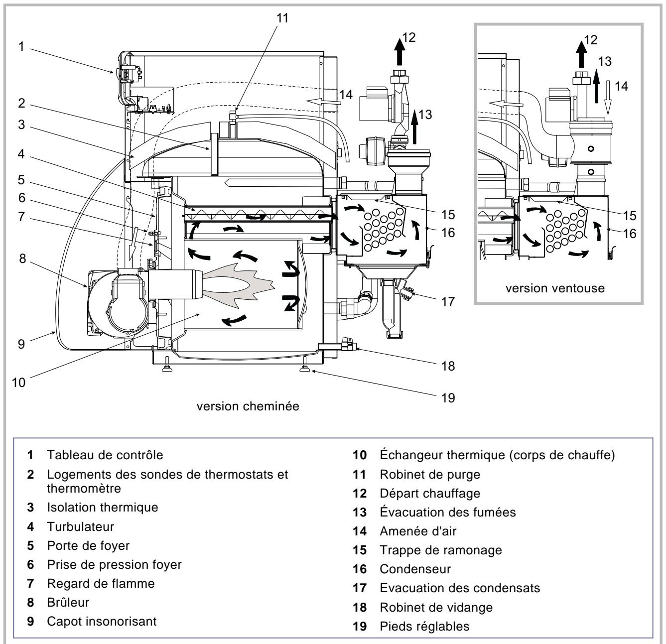
Figure 10 - Coupe schématique de l'appareil
