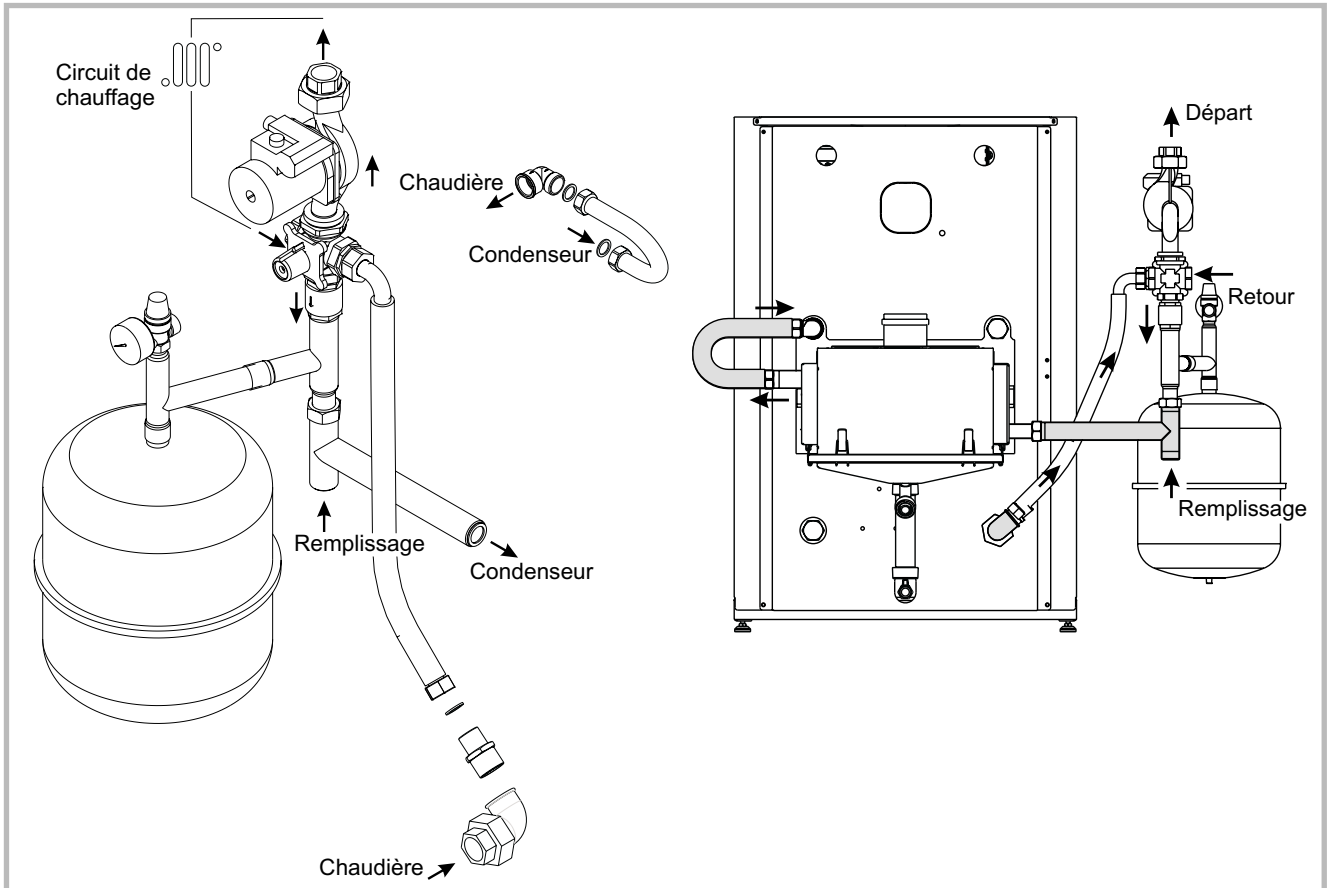
Figure 21 - Montage du kit hydraulique
