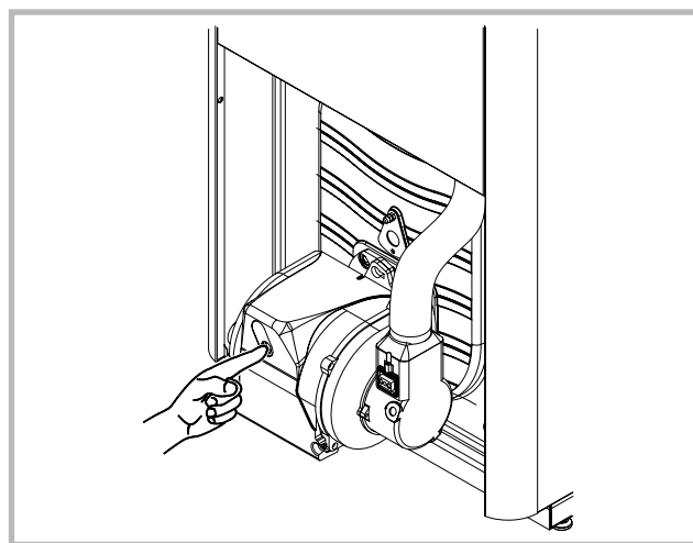
Figure 42 - Touche de réarmement (sécurité du brûleur)
