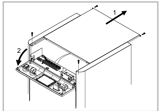
Figure 29 - Accès aux bornes de raccordement
