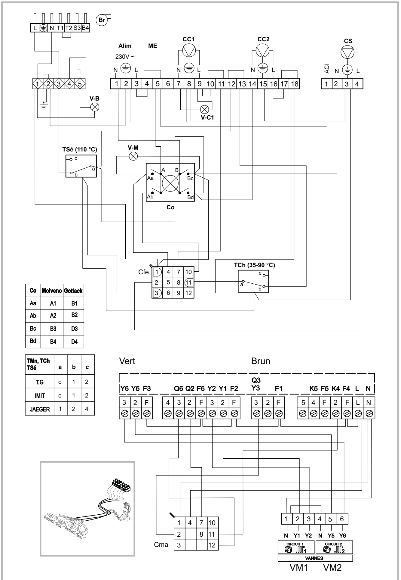
Figure 32 - Câblage électrique (Chaudière)
