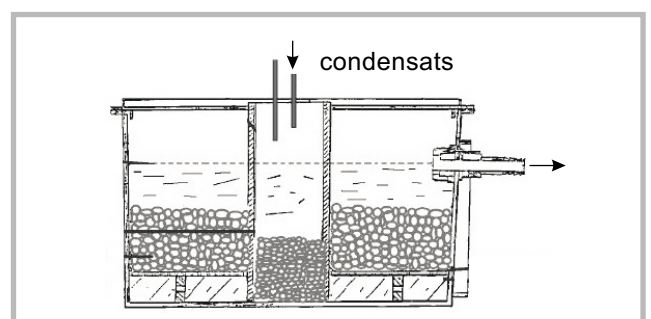
Figure 18 - Bac de neutralisation
