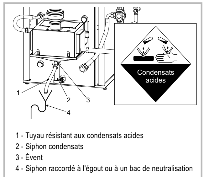
Figure 17 - Évacuation des condensats
