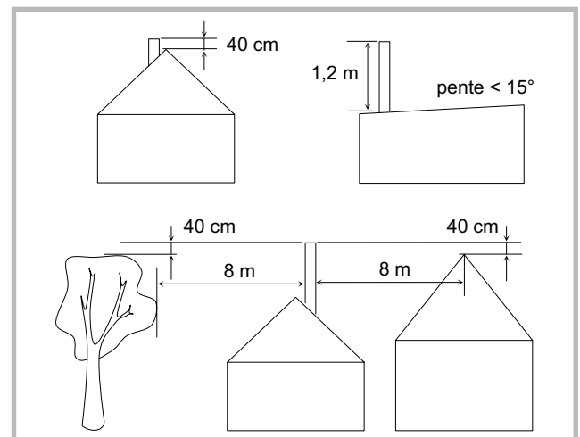
Figure 12 - Hauteur de la souche du conduit d'évacuation (B23P)
