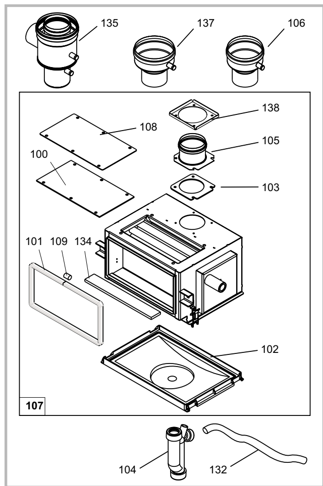
Figure 45 - Vue éclatée (condenseur)
