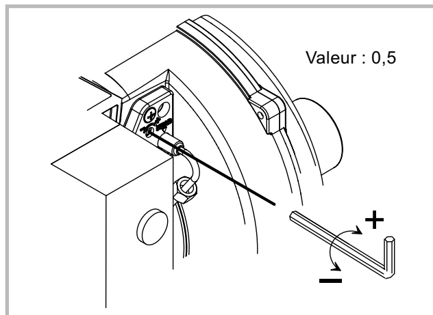
Figure 33 - Réglage de la tête de combustion
