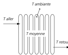
E60 = la puissance d'émission lorsque T moyenne - T ambiante = 60°C
